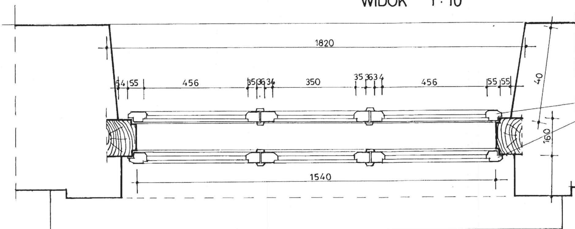
RZUT 1:10
