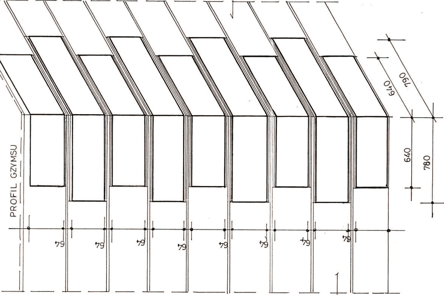
NAROŻNIK OFICYNY PROFILE BONIOWANIA 1:20
