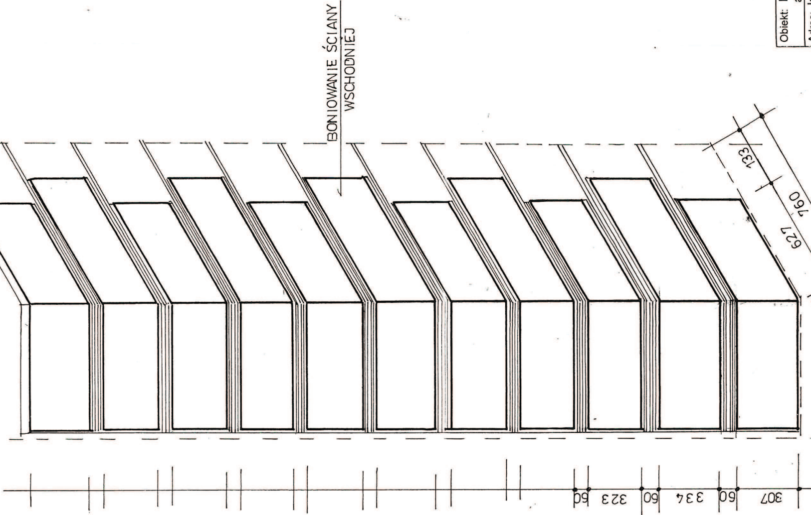
NAROŻNIK LEWY KORPUS GŁ. STRONA WSCHODNIA 1:20
