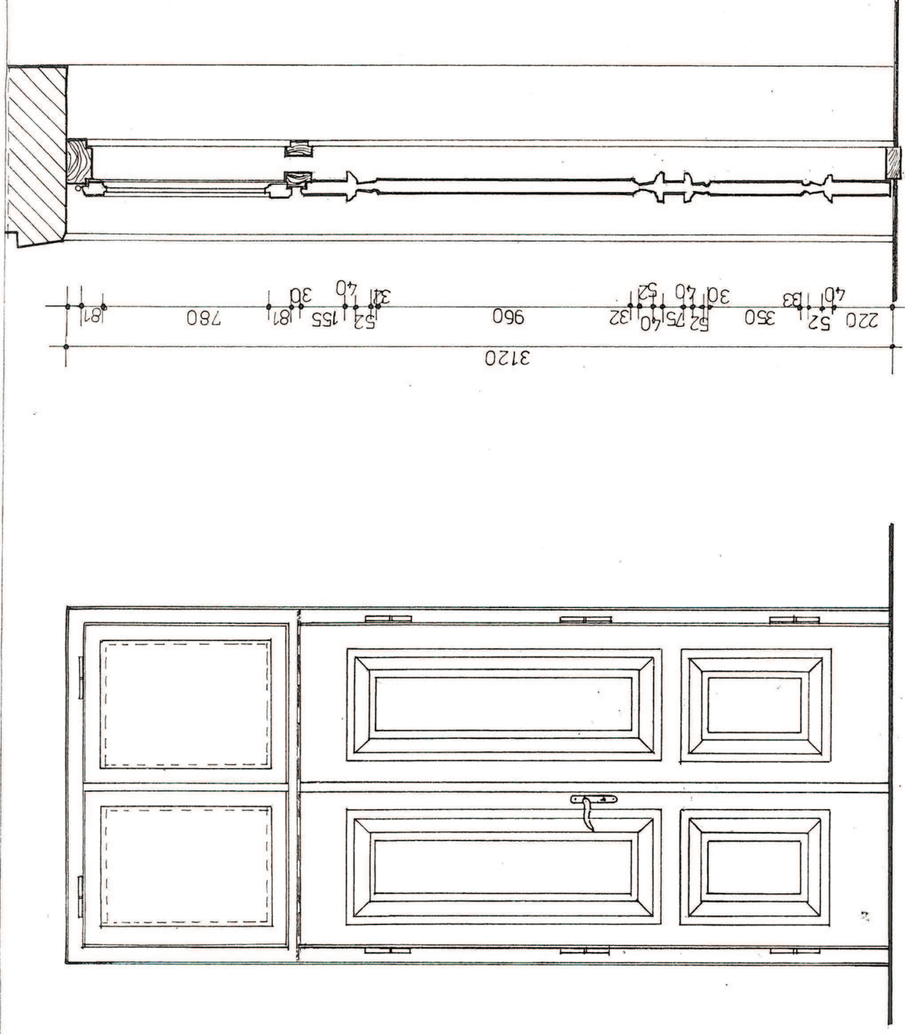
WIDOK 1:20
