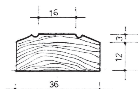
LISTWA 1:1
