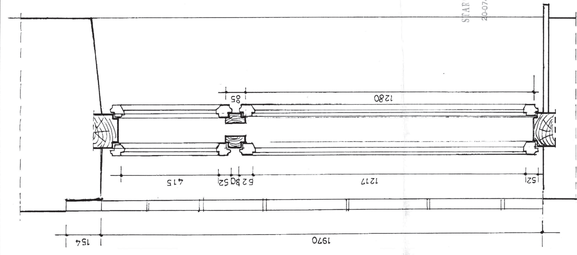
PRZĘKŁÓJ A-A 1 : 10
