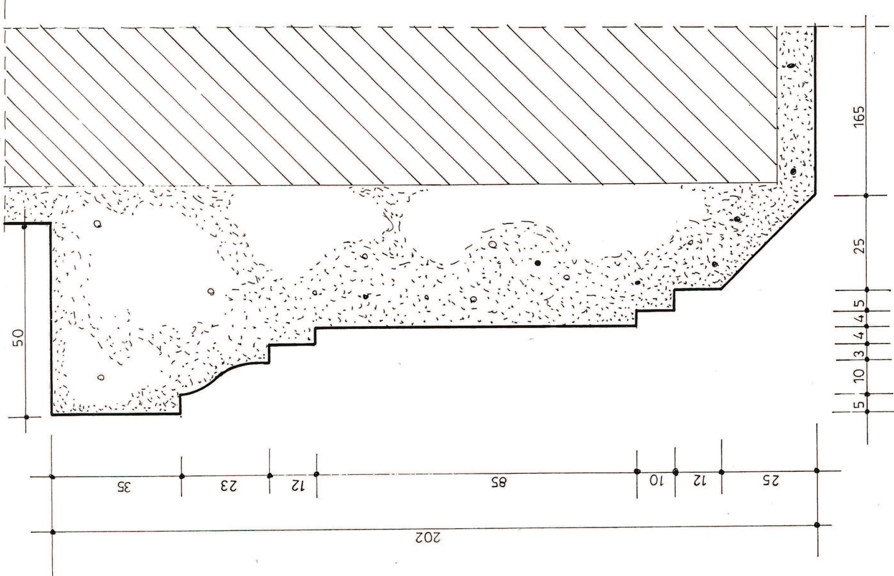
PROFIL OPASKI OKIENNEJ 1:1 A-A OFICYNA POŁUDNIOWA - PARTER
