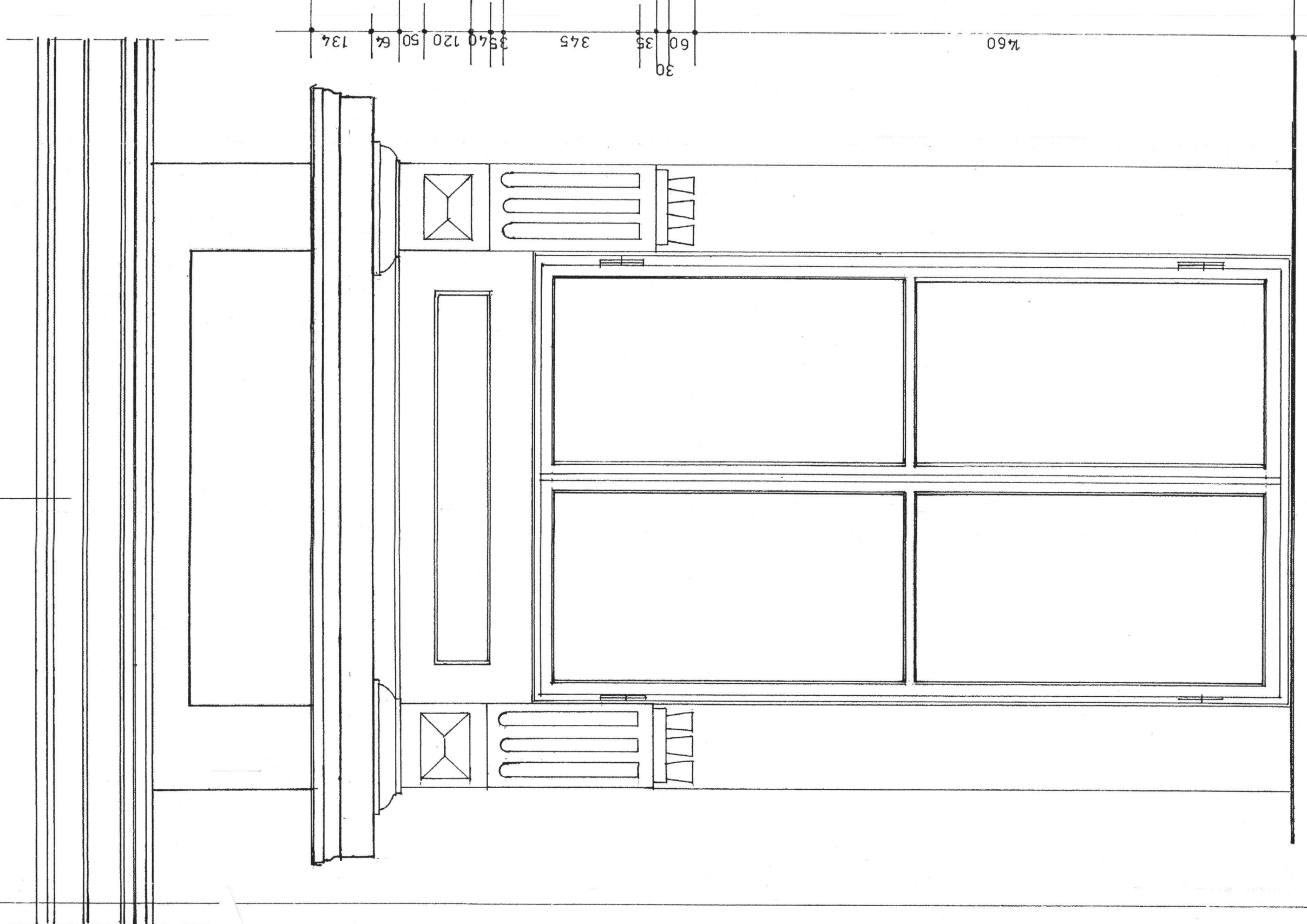
OPRAWA OKNA 1:10
