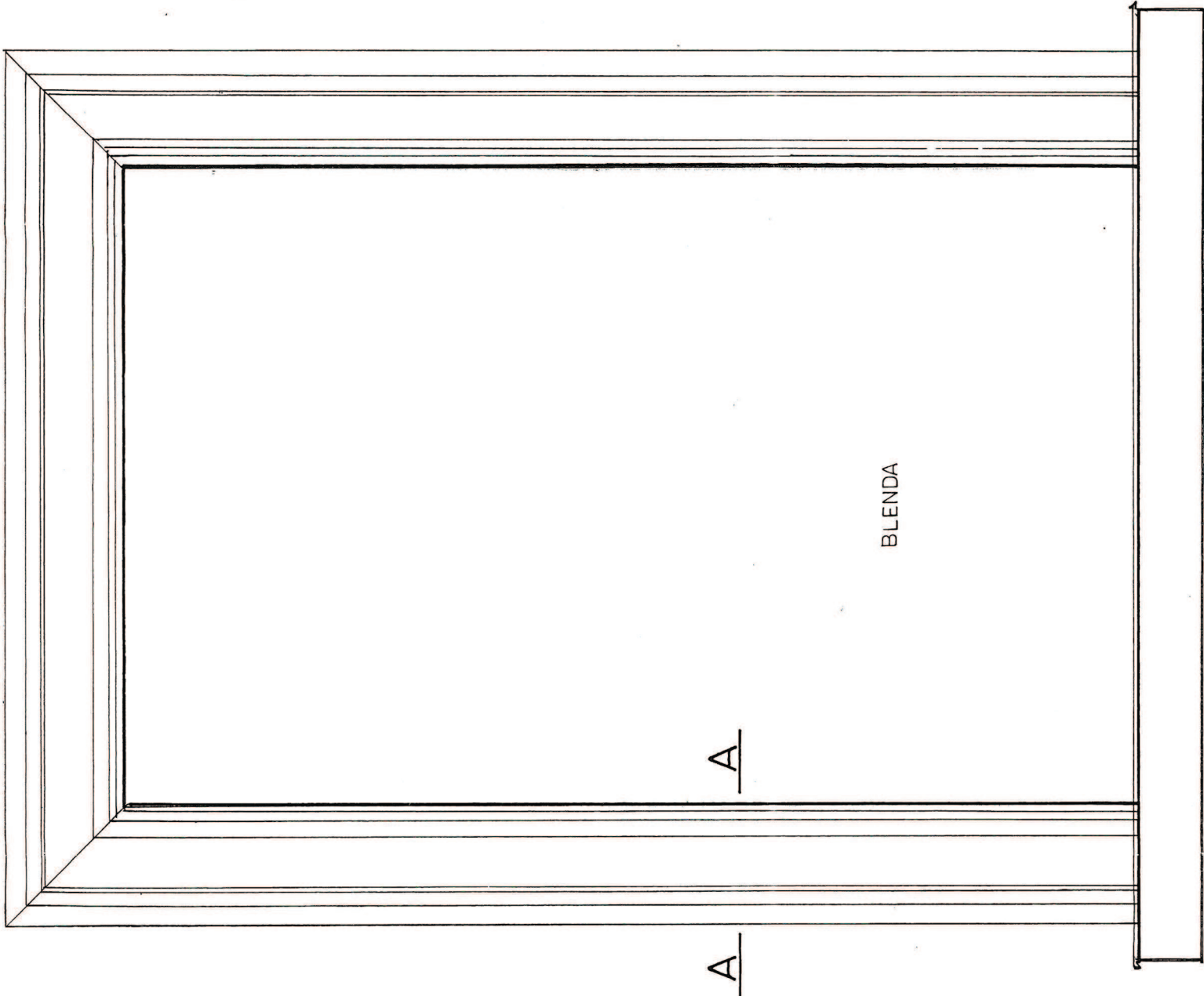
OPRAWA BLENDY 1:10
