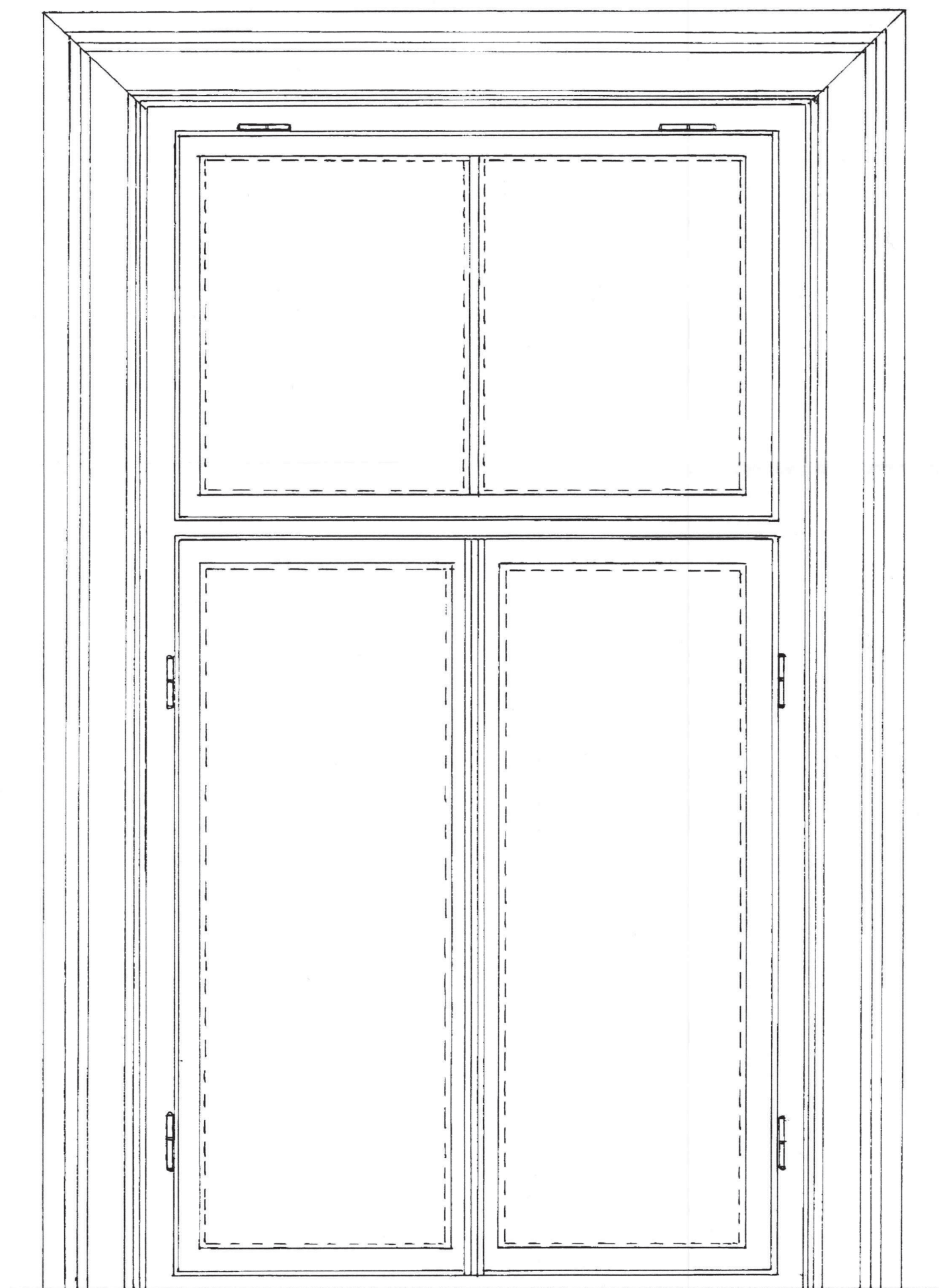
WIDOK 1:10
