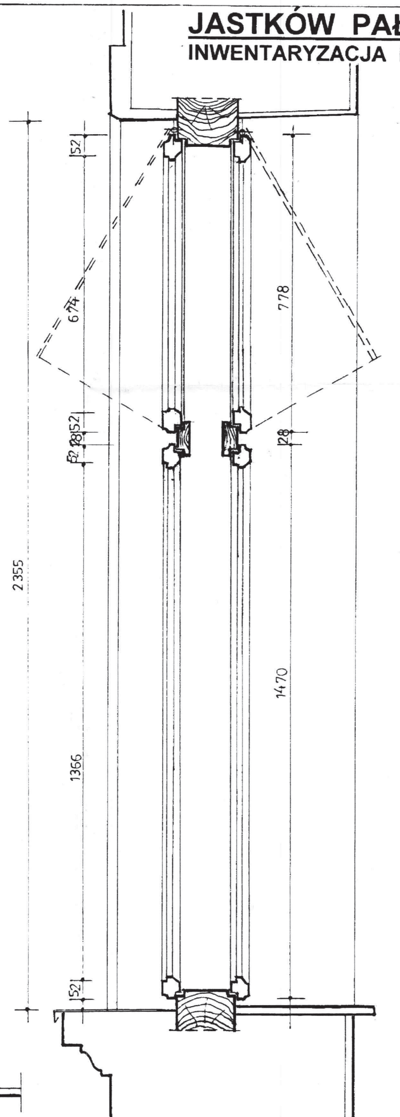
PRZEKRÓJ A-A 1:10
