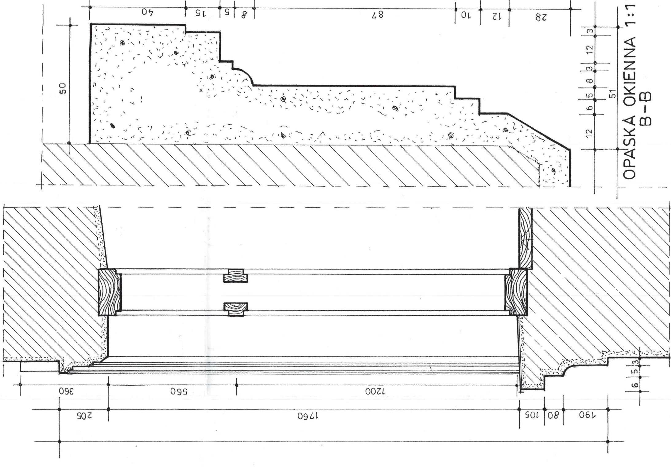
PRZEKRÓJ PIONOWY 1:10 A-A
