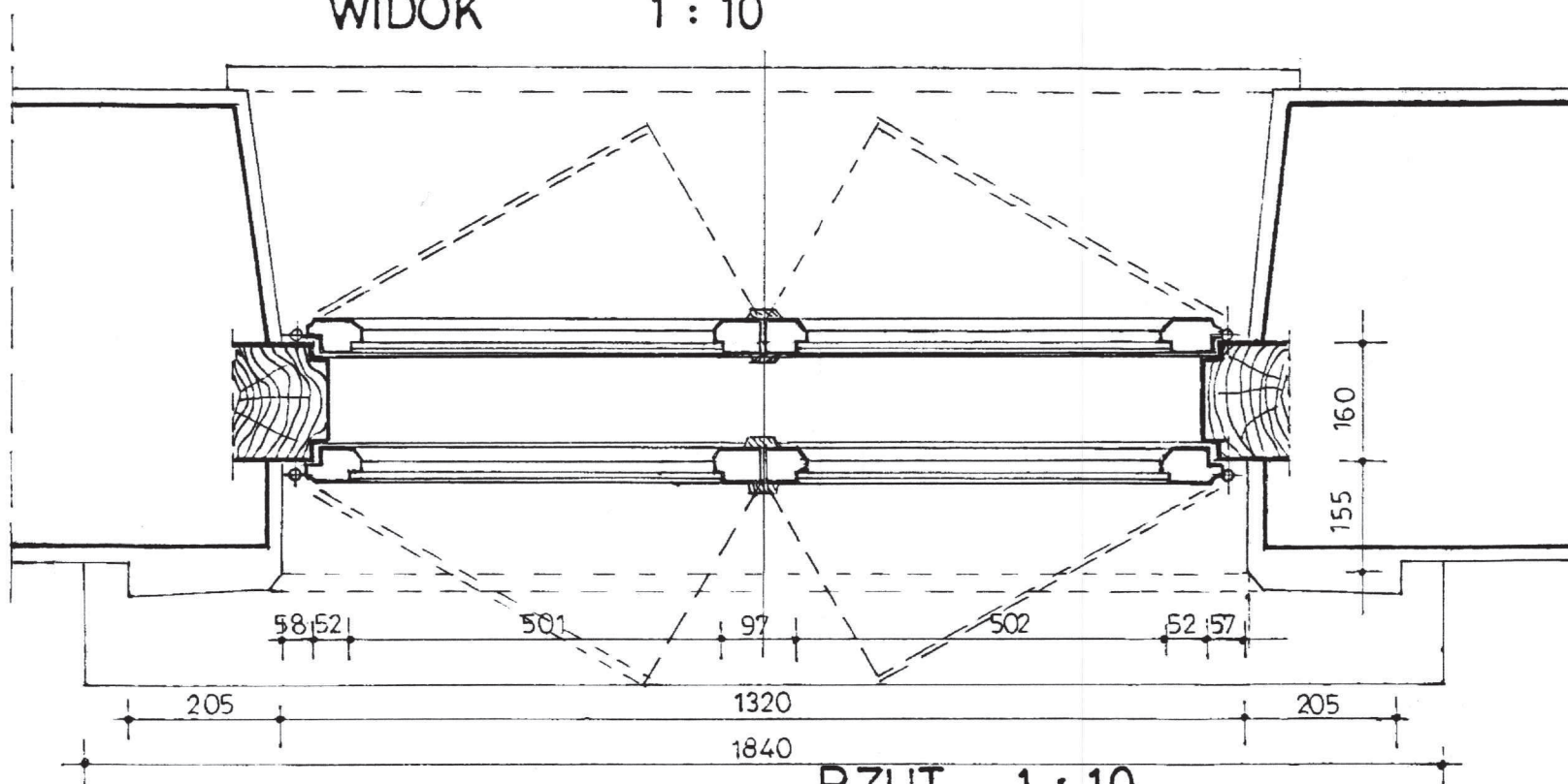
RZUT 1:10
