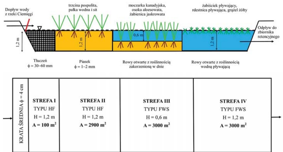
Rysunek 1. Schemat technologiczny systemu hydrofitowego do oczyszczania wód powierzchniowych z rzeki Ciemięgi
